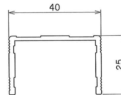
支柱
