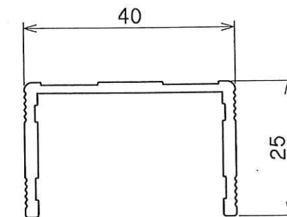
支柱
