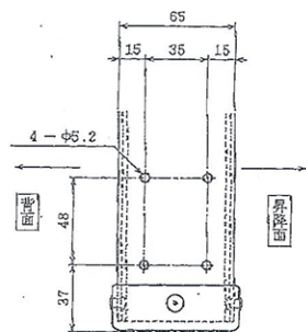
支柱穴加工図
