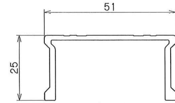
支柱(1/1)
