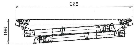
収納状態
