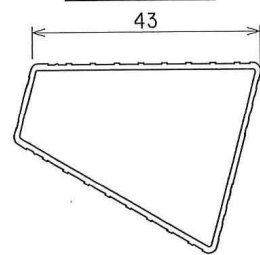
踏ざん(1/1)
