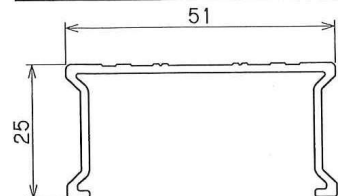
支柱(1/1)
