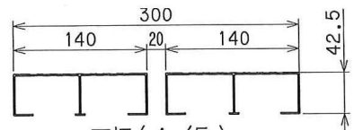
天板(1/5)
