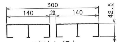
天板(1/5)
