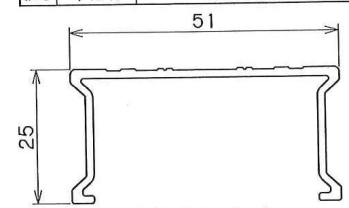
支柱(1/1)
