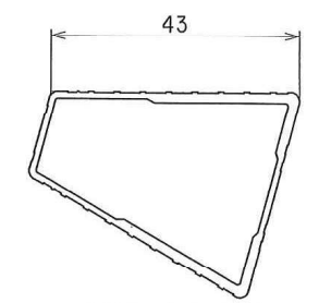
踏ざん(1/1)
