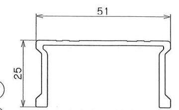
支柱(1/1)
