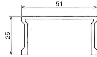
支柱断面図 (1/1)
