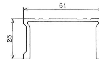
支柱断面図 (1/1)
