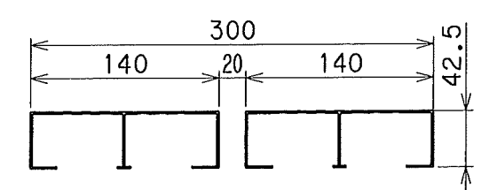
天板 (1/5)
