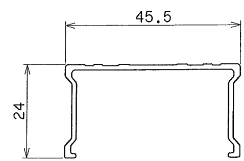
支柱 (1/1)
