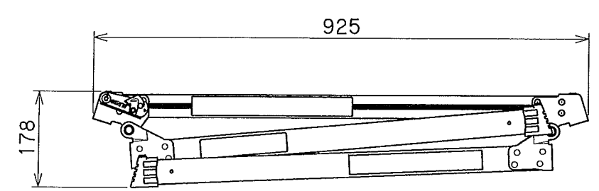
収納状態
