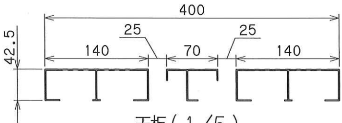
天板(1/5)
