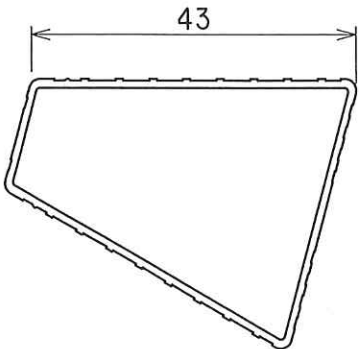
踏ざん(1/1)
