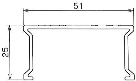
支柱(1/1)
