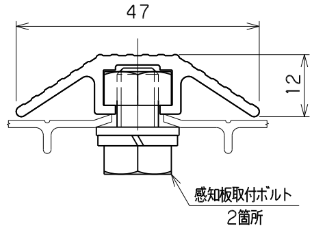
妻面感知板取付図 ( 1 / 1 )
