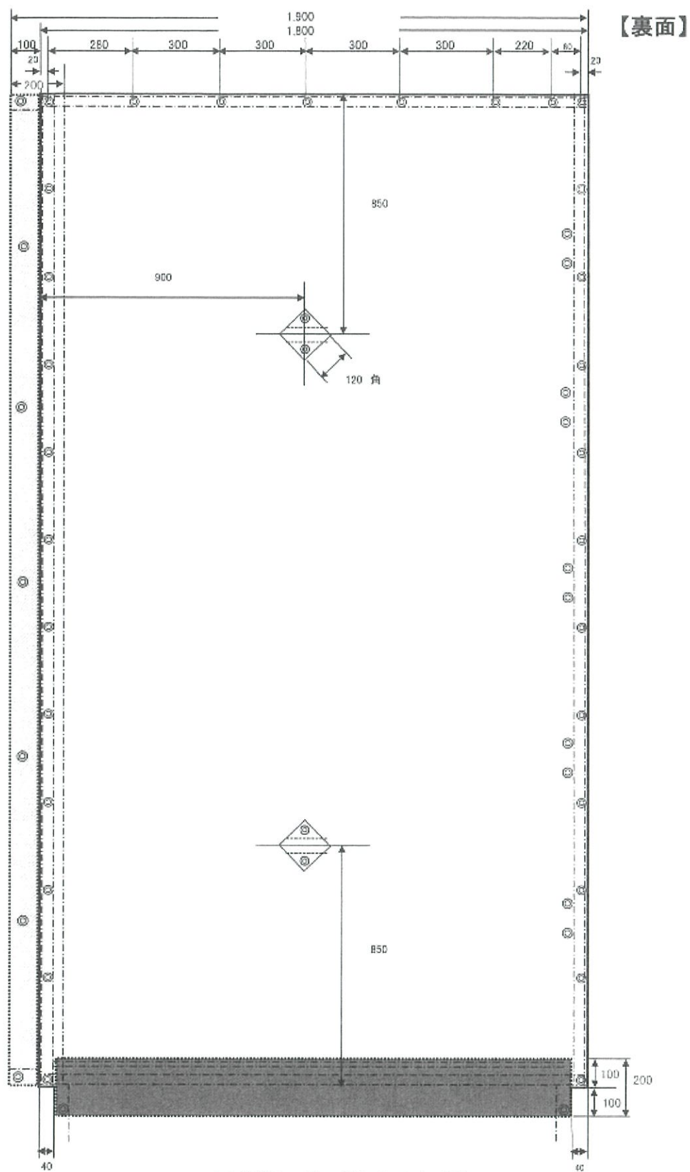
加工仕様図 新工口防音1.8×3.4 【裏】
