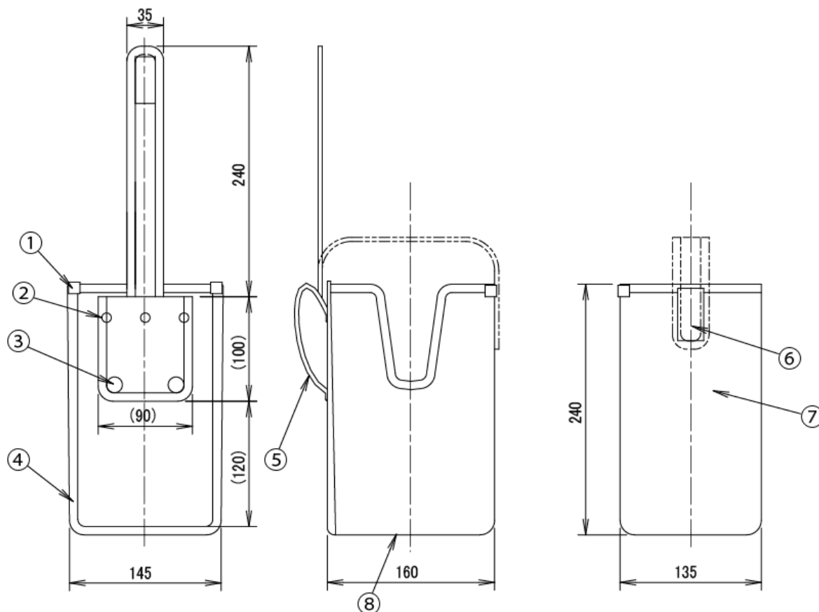
○外觀寸法図
