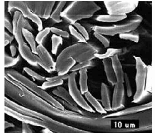
超細分割繊維<WRAMP>の繊維構造 (電子顕微鏡写真)
