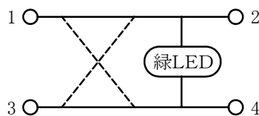
内部回路図
