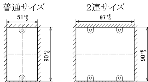
加工穴寸法(単位mm)
