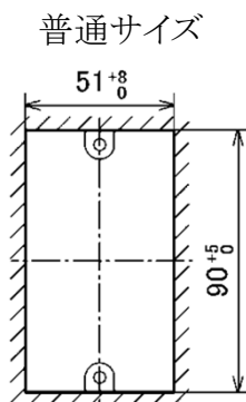
加工穴寸法 (単位mm)
