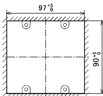
加工穴寸法(単位mm)
