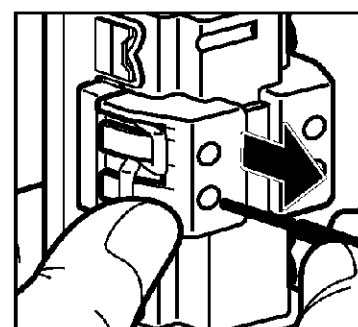
③電線を引き抜く
