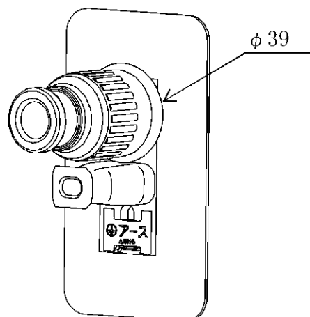
φ 39 接地防水ゴムキャップ1 個と 平形キャップ1 個
