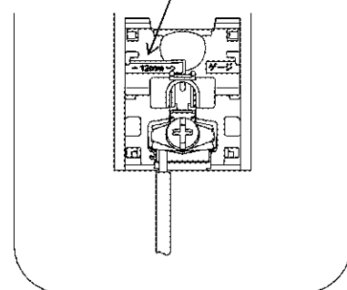
ストリップゲージ
