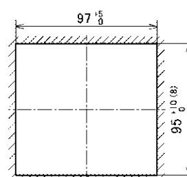
加工穴寸法(単位mm)
