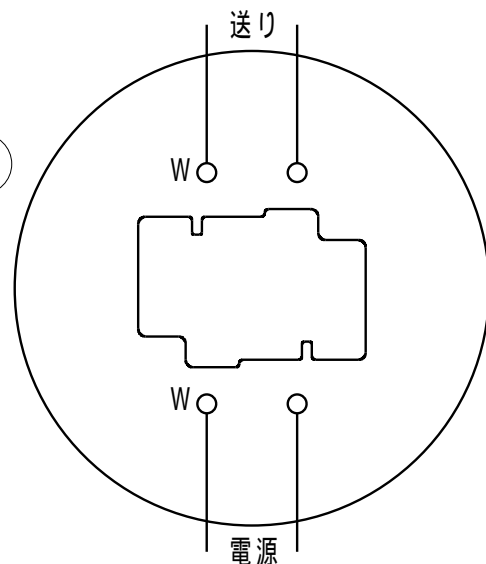
結線図（裏面図）
