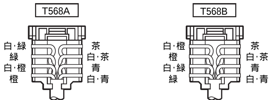
結線図
