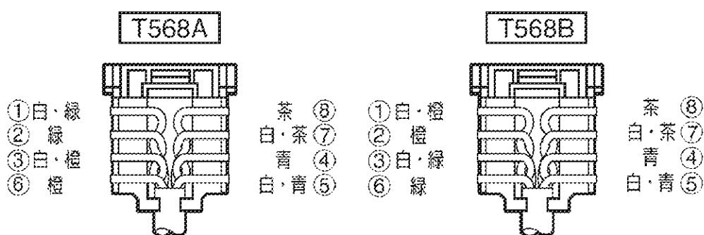
結線図
