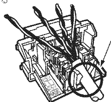
ケーブル 固定部
