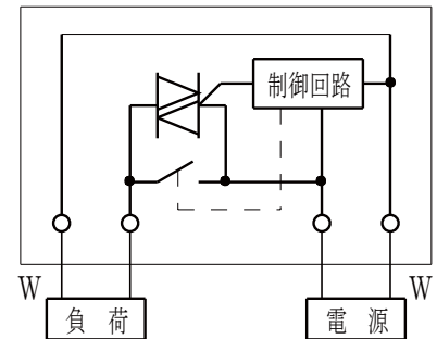
内部回路図
