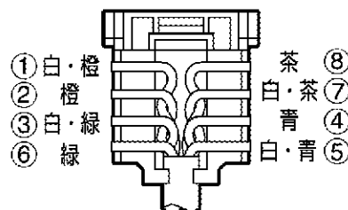
結線図
