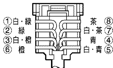
T568A
