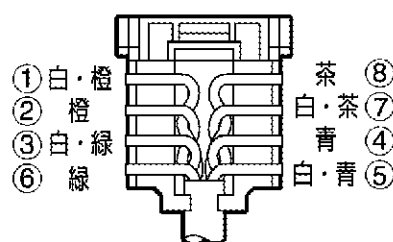
結線図
