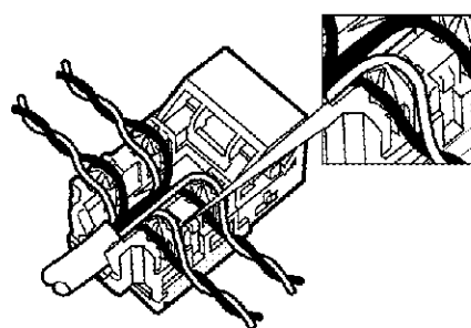
T568A
