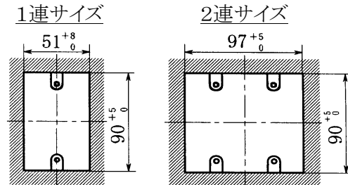
加工穴寸法(単位mm)
