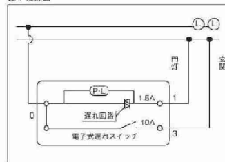
標準結線図
