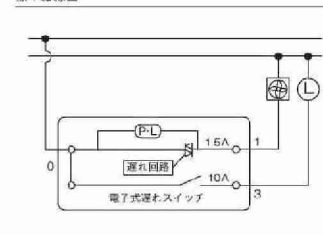
標準結線図
