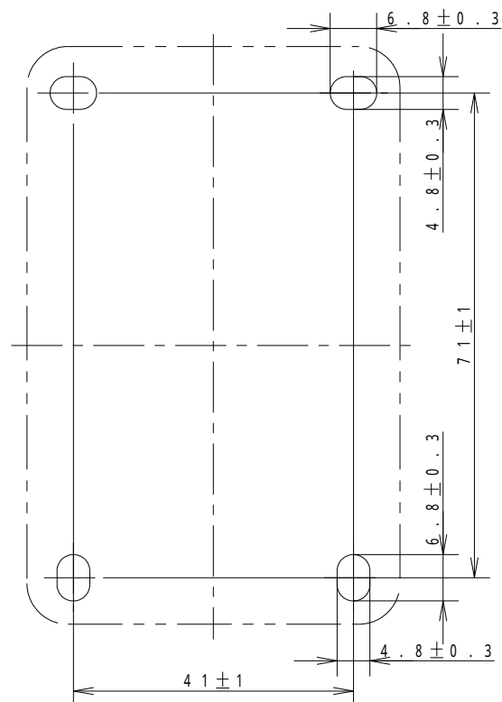
取付寸法
