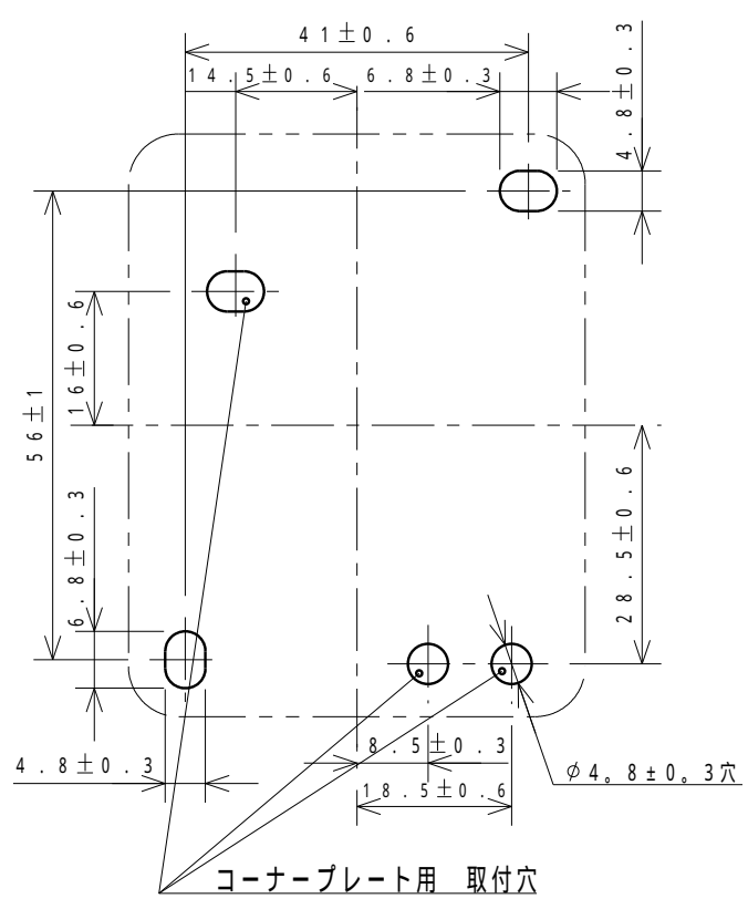
取付寸法
