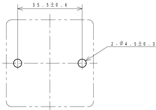
取付寸法
