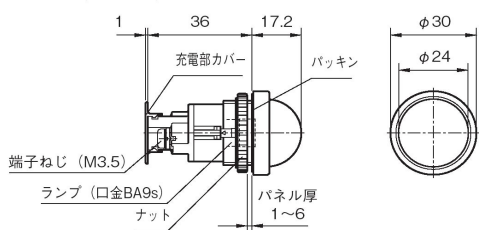
〔全電圧式〕 EA940DB-91～-94
