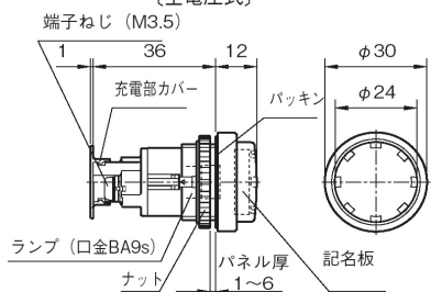
〔全電圧式〕 EA940DB-106～-109
