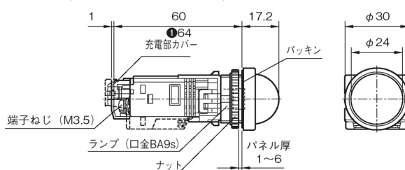
〔トランス・抵抗ユニット式〕 EA940DB-96～-104
