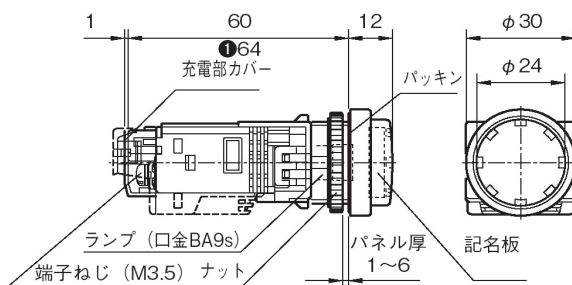
〔トランス・抵抗ユニット式〕 EA940DB-111～-119
