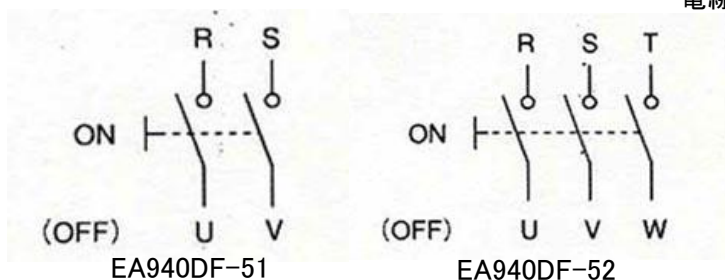
(接点構成表)
