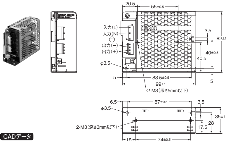
取り付け穴加工寸法
