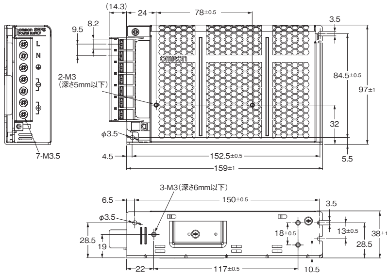
取り付け穴加工寸法
