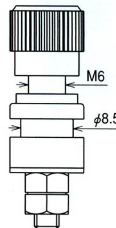
取付孔寸法例
