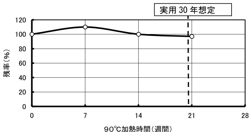
図 2. 接着耐久性
