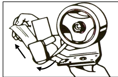
② ローラーとテープ押さえの間からテープを引出します。
