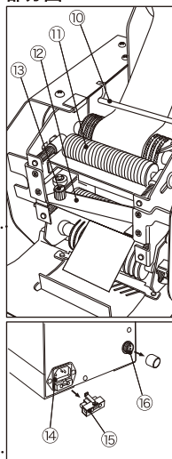
部分図
