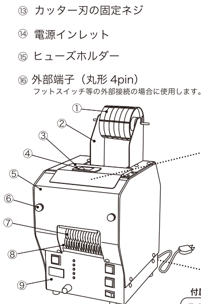
部分図
