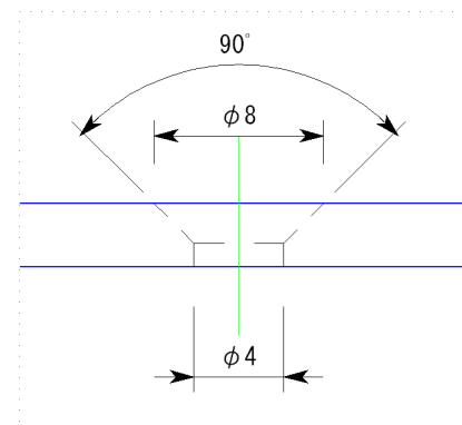
皿加工部詳細
