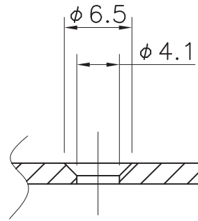
A部拡大図 (S=2:1)
