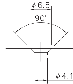
A部拡大図(S=2:1)
