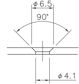
A部拡大図 (S=2:1)
