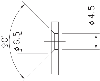
A部拡大図(S=2:1)
