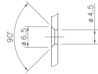
A-A矢視図(S=2:1)
