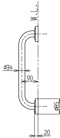
取付座詳細(1:2)
