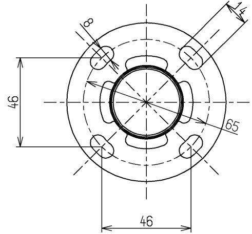
取付座詳細(1:2)
