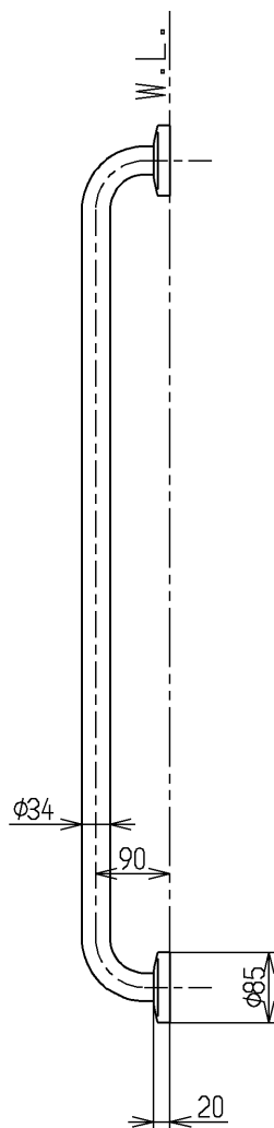
取付座詳細(1:2)
