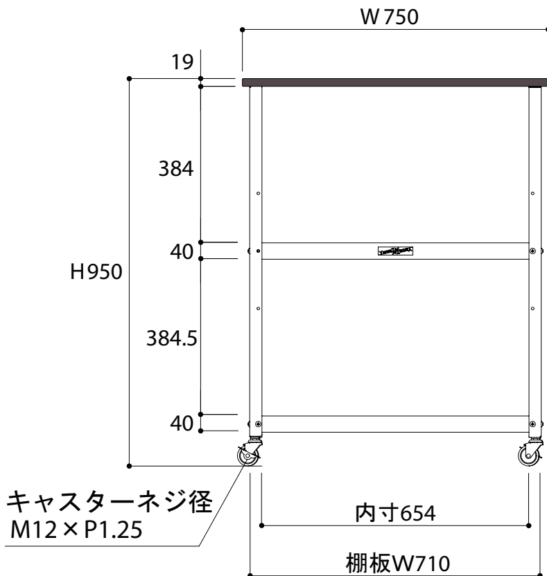
正面図
