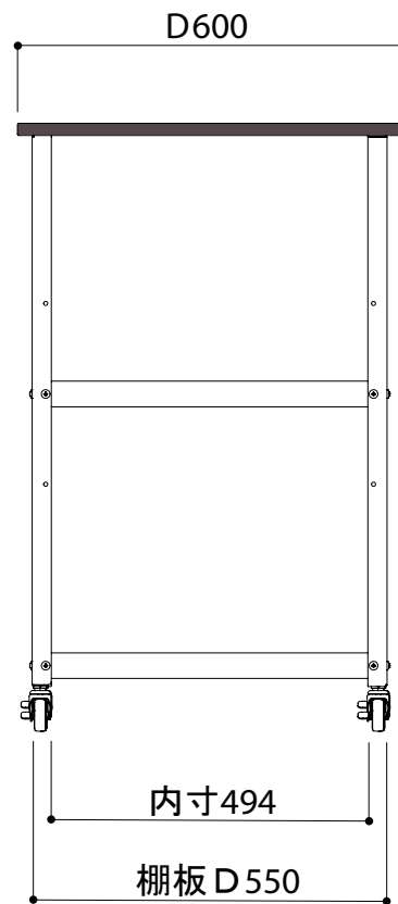
側面図
